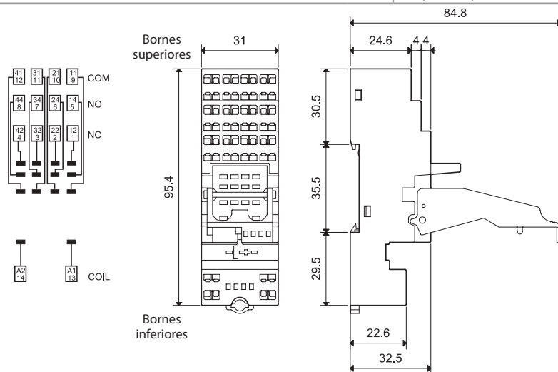
Zócalo + Puente
